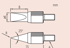
Knife edge point
