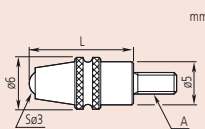
Ball point (21AZA320)
