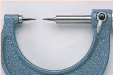
Tip angle : 15°
