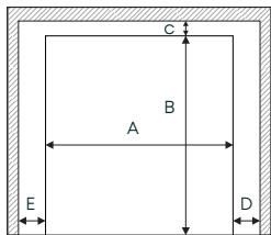
Calha Padieira Reduzida (Molas Recuadas)
