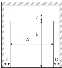
Calha Inclinada Dupla / Simples
