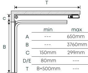
Calha Inclinada Dupla / Simples
