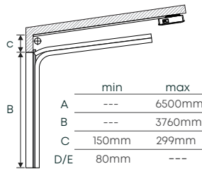
Calha Inclinada Dupla / Simples
