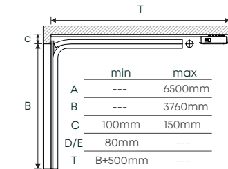
Calha Padieira Reduzida (Molas Recuadas)
